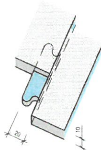
Detail "Schwalbenschwanz"
